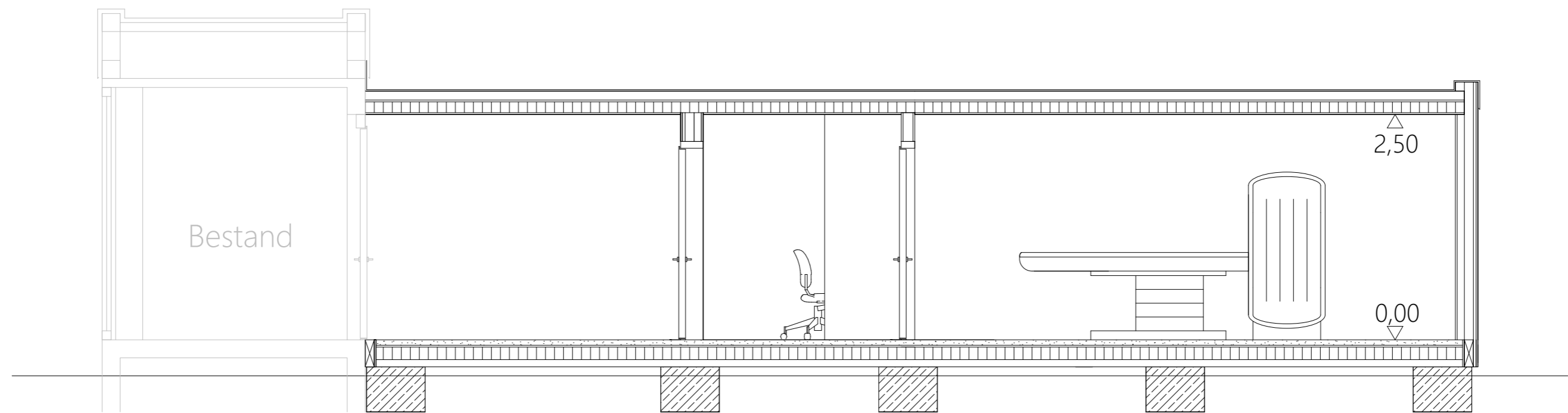
Schnitt A
